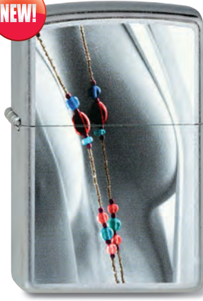
Hot Rod 2.003.114 #207 · 39,95 €
