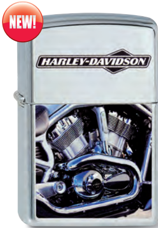
H-D® Engine 2.003.092 #250 · 46,95 €
