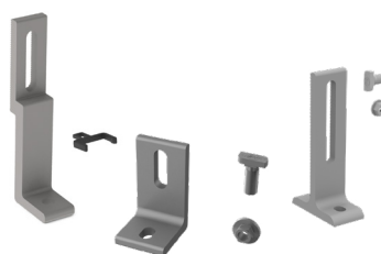
L-Foot & T-Foot
