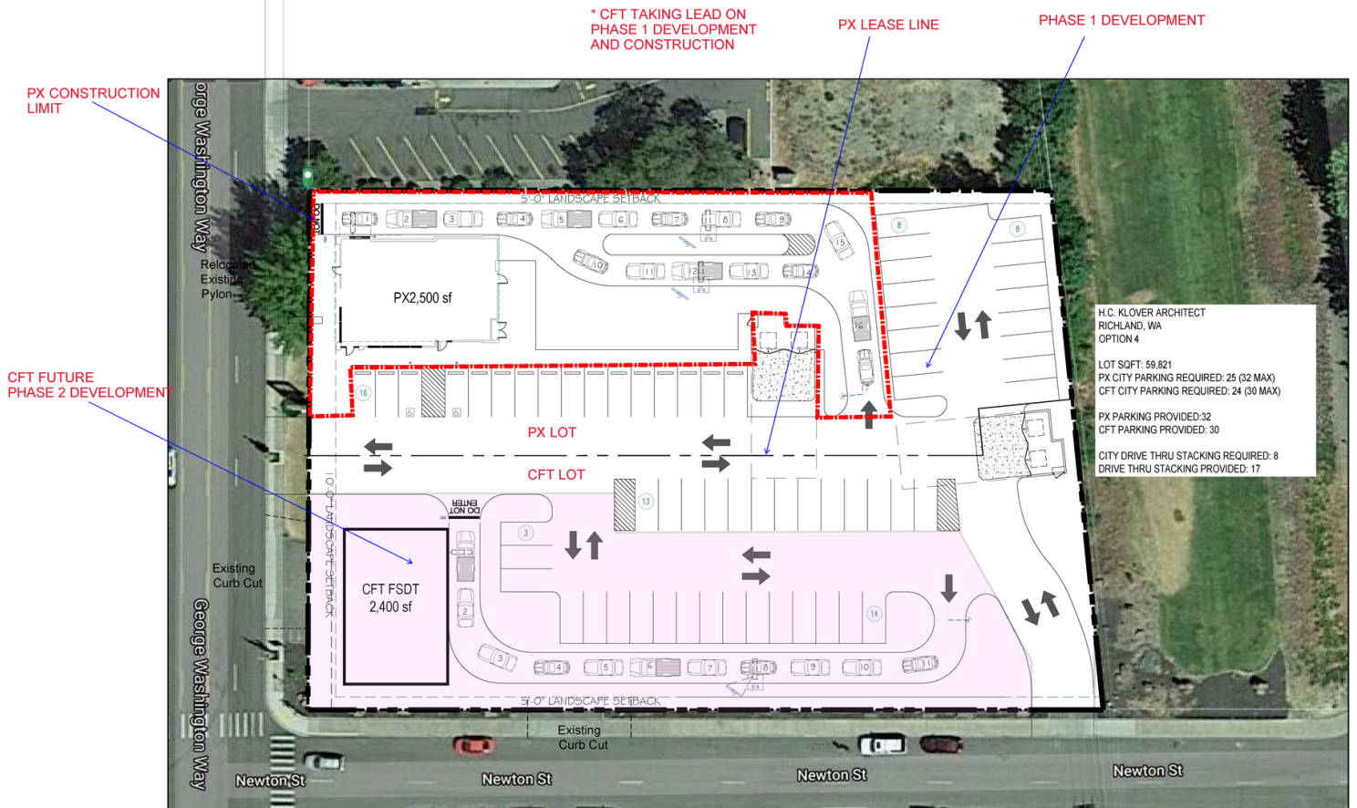
SITE PLAN - OPTION 4.1
