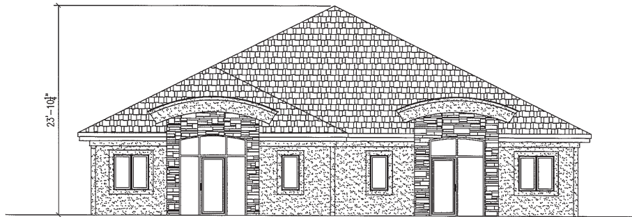
FRONT ELEVATION SCALE: 1/8"=1'-0"
