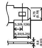
F1 (FASTON TAB NO. 187)
