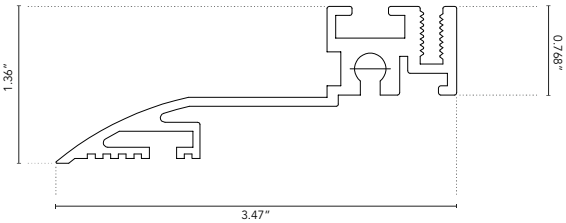
Edge profile
