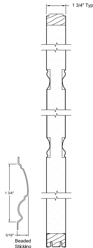
Section A-A
