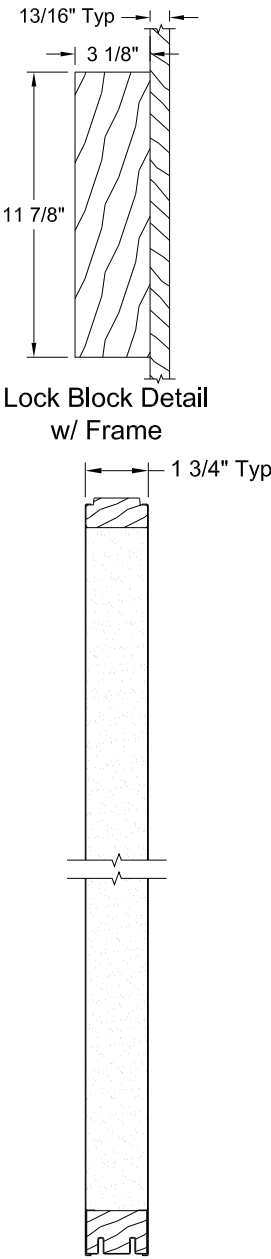
Section A-A
