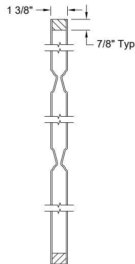
Section A-A Ovolo Sticking
