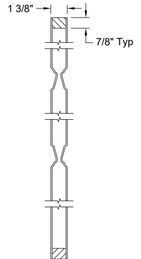
Section A-A Ovolo Sticking
