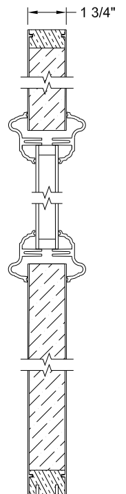
Section A-A
