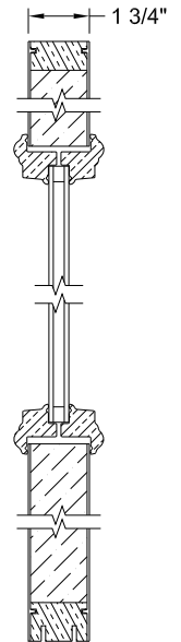
Section A-A
