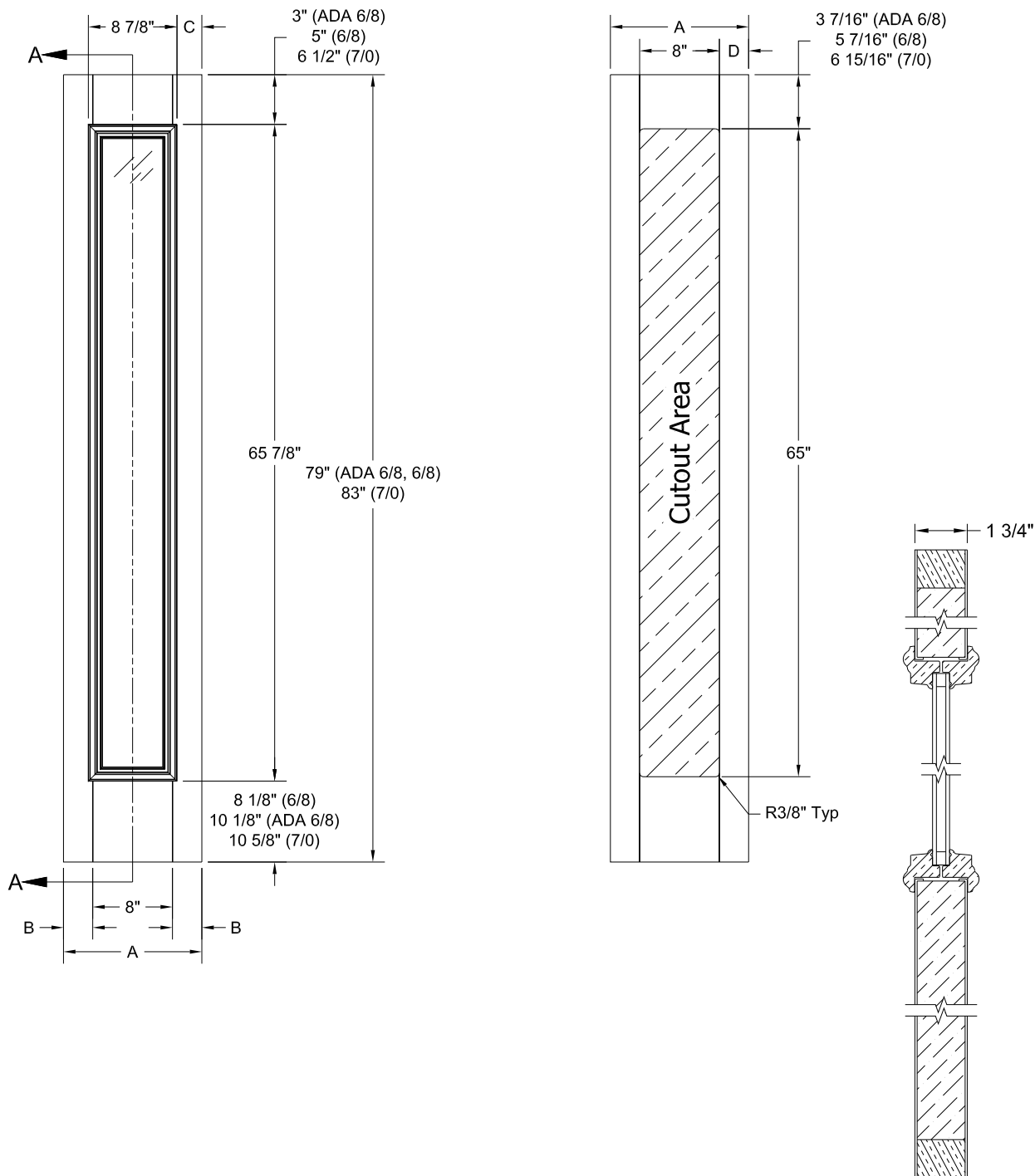
Section A-A
