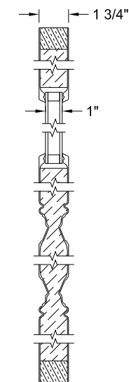
Section A-A
