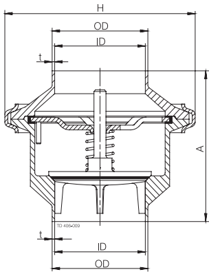
Fig. 4. Dimensions
