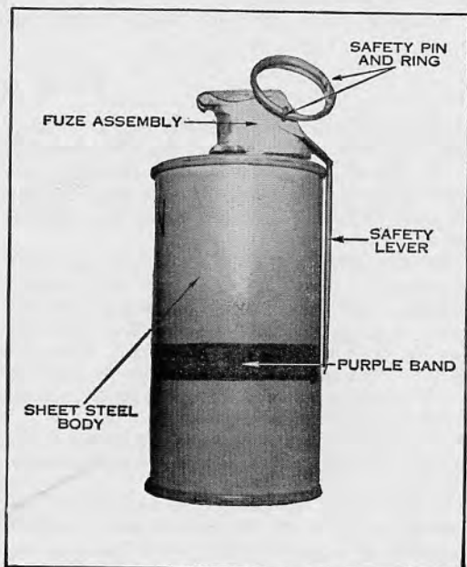
25.4 Incendiary Grenade AN-M14.
