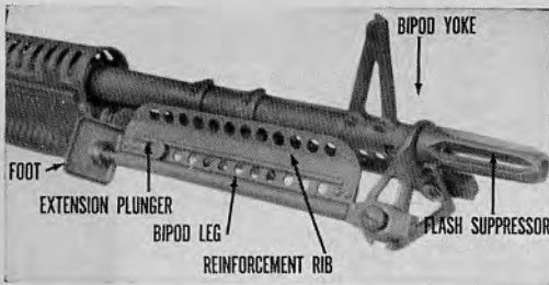
36.34(a) Bipod mount.
